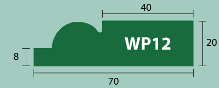
Torus Architrave
